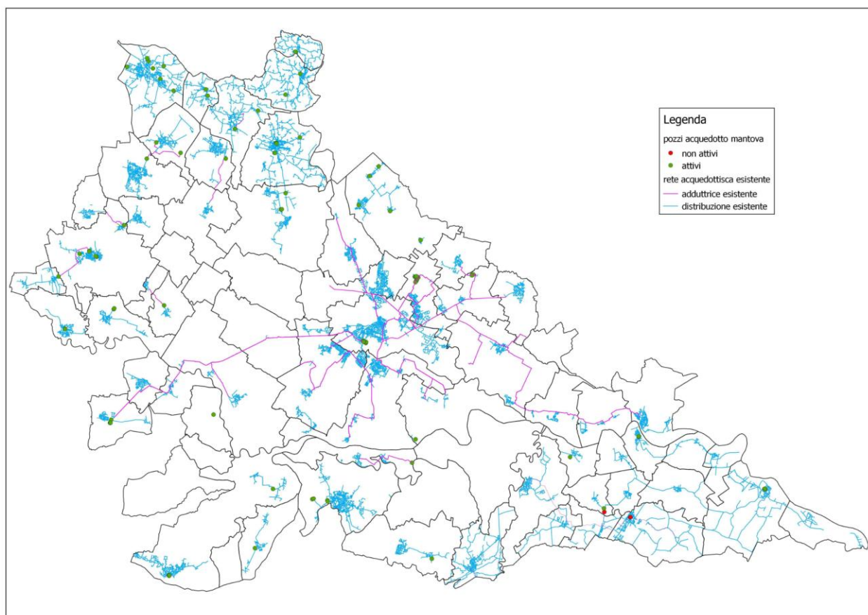
Rete acquedotto
